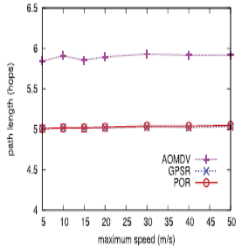
(d) Path length.
