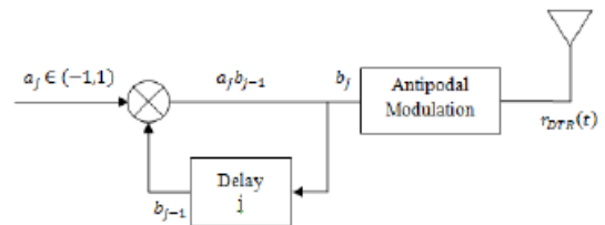
Fig. 1. DTR Transmitter
